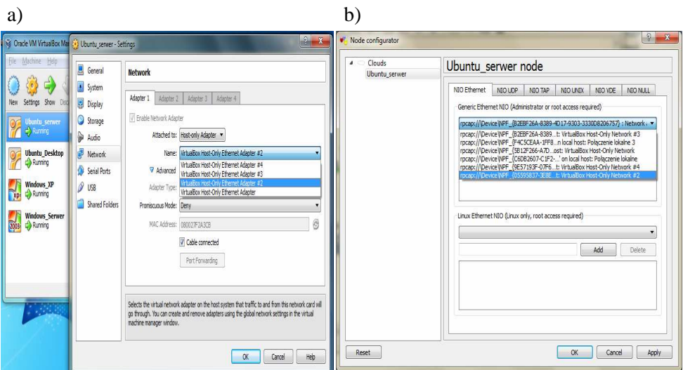
Rys. 3. Opcje dowiązania jednego z interfejsów wirtualnych: a) do maszyny wirtualnej, b) do odpowiadającego jej węzła w GNS3
