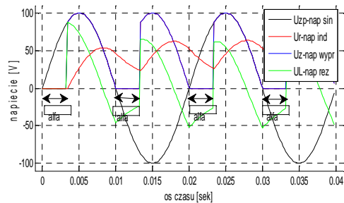
Rys. 5. Sygnały napięć dla układu prostowniczego dwupołówkowego dla danych: U_m = 100[V] , R = 20[\Omega] , L = 0.1[H] , f = 50[Hz]
