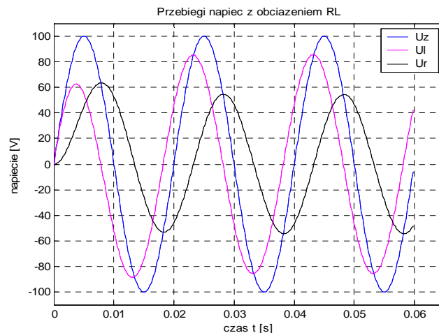
Rys. 2. Sygnały napięć w obwodzie dla danych: U_m = 100 , R = 10 , L = .05 , f = 50
