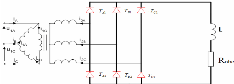
Rys. 6. Schemat układu prostowniczego trójfazowego
